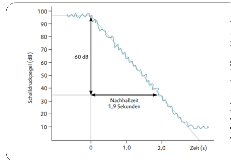
Nachhallzeit in Sekunden (s) nach Schalldruckpegel (dB)
