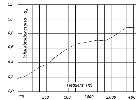
Schallabsorptionsgrad – Oktav-Mittenfrequenz
