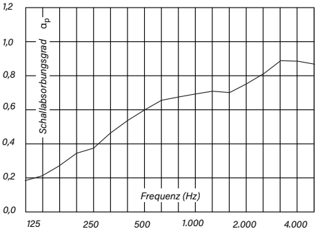
Schallabsorptionsgrad – Oktav-Mittenfrequenz
