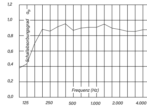
Schallabsorptionsgrad – Oktav-Mittenfrequenz
