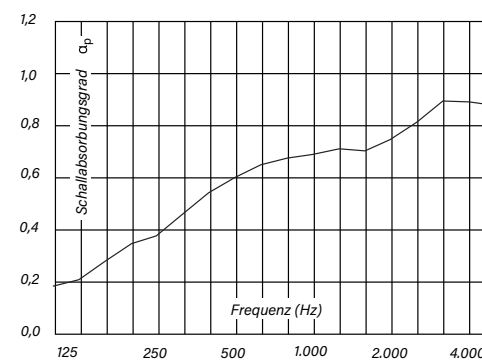
Schallabsorptionsgrad – Oktav-Mittenfrequenz
