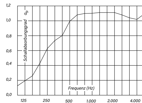
Wandabsorber 40 mit Wechselbezug
