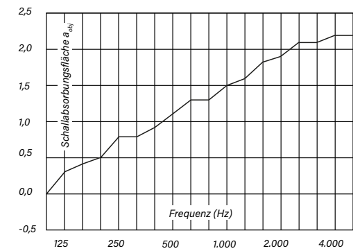
Äquivalente Schallabsorptionsleistung A_{obj}
