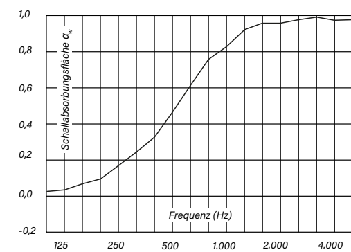
Schallabsorptionsgrad – Oktav-Mittenfrequenz
