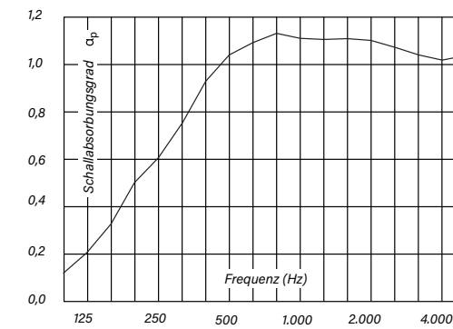
Schallabsorptionsgrad – Oktav-Mittenfrequenz (Würfel)
