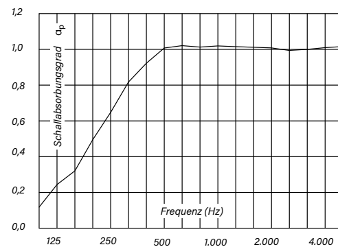
Schallabsorptionsgrad - Oktav-Mittenfrequenz
