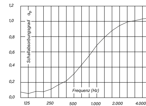
Schallabsorptionsgrad – Oktav-Mittenfrequenz
